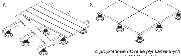
1. przykładowe ułożenie tarasu z legarami na wspornikach DD Pedestals
